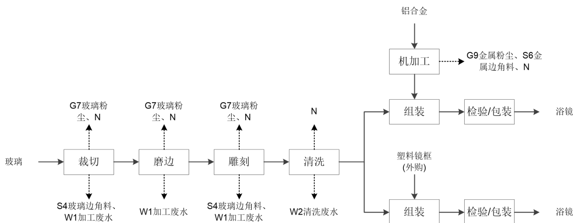
图 4 浴镜生产工艺流程图
