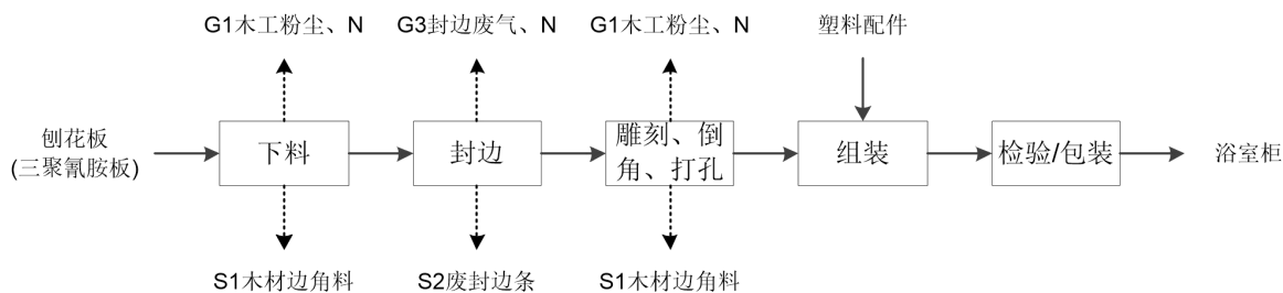
图 2 浴室柜产品生产工艺流程图
